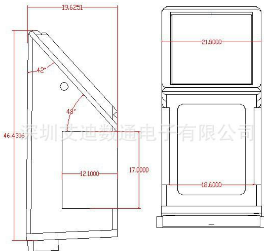
图2-1 A32尺寸图
